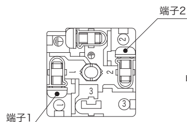
DIN连接器端子配置
