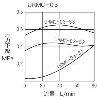
压力下降特性
