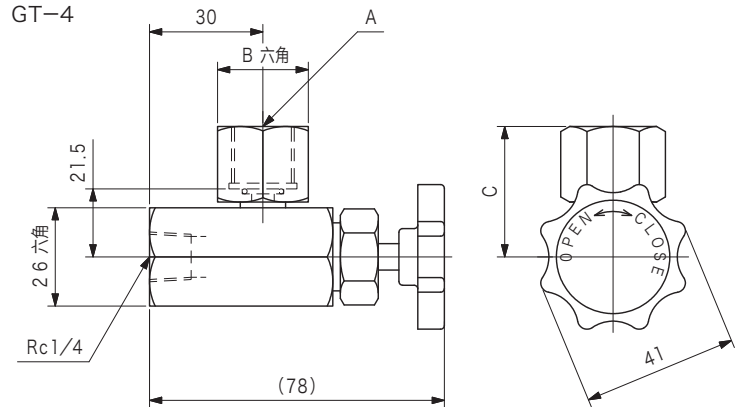
尺寸表
