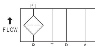
液压图形符号
